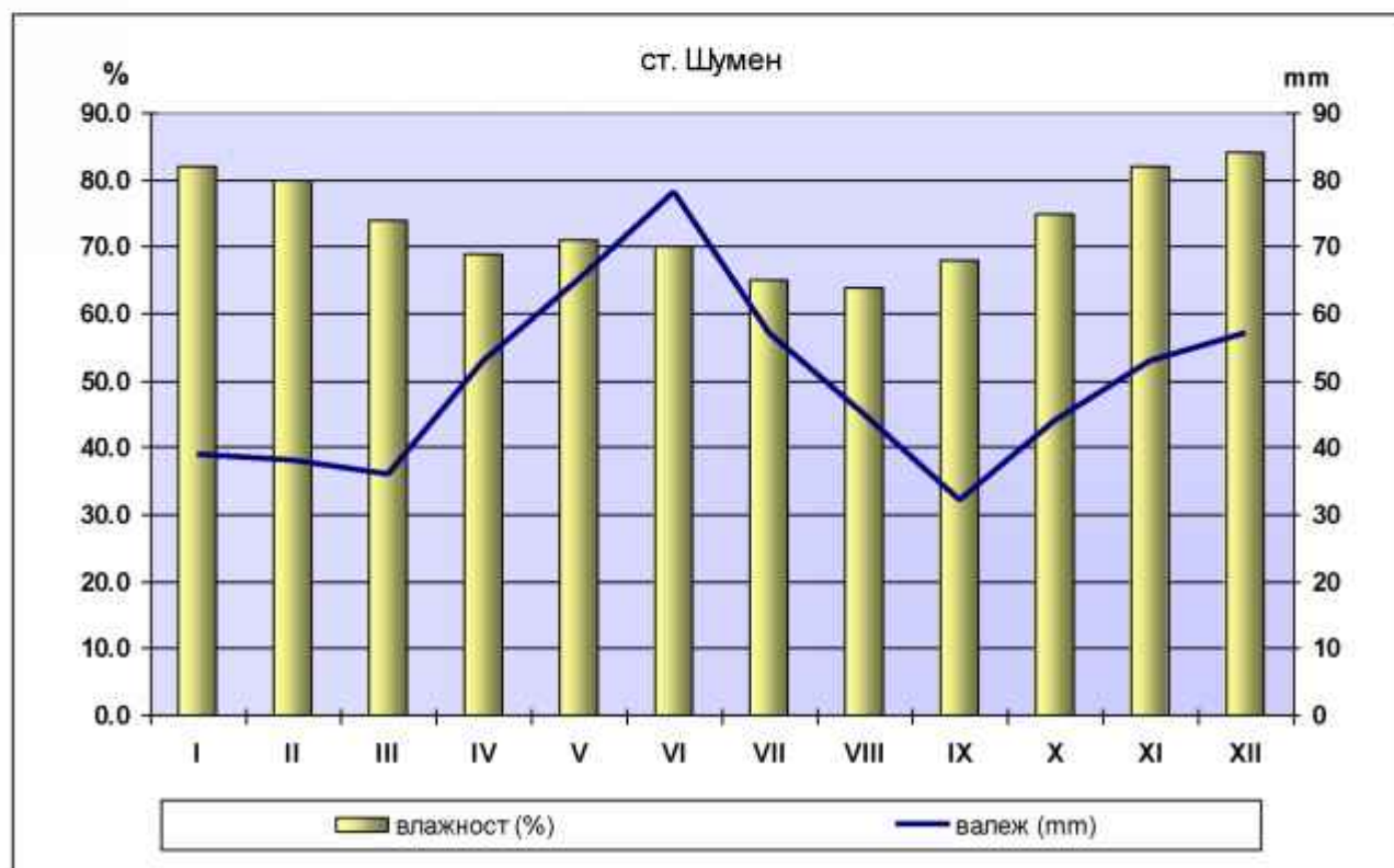
Фиг. 4.а -3. Годишен ход на средномесечните валежи и относителната влажност за гр. Шумен
